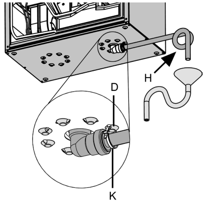
Abbildung: Lüftungsgerät in Rechtsausführung, Linksausführungen spiegelt
